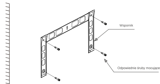
Rysunek 5.4 Montaż falownika na ścianie
