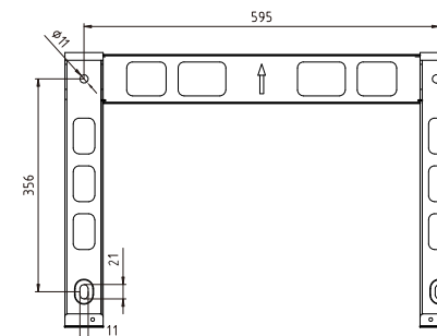
Rysunek 5.3 Montaż falownika na ścianie
