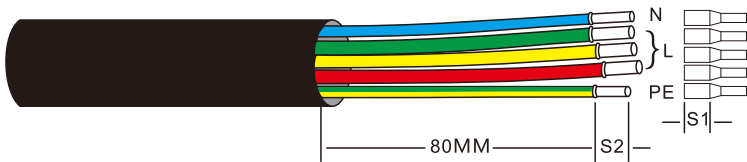
Rysunek 5.23 Zdjęcie izolacji z kabla prądu zmiennego
