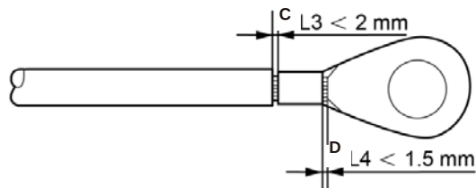
Rysunek 5.13 Przewód ze zdjętą izolacją
