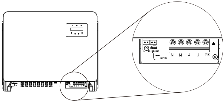
Rysunek 5.24 Okablowanie
