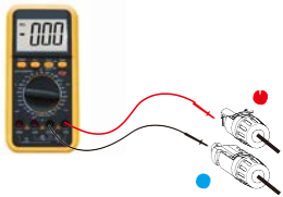
Rysunek 5.21 Pomiar z użyciem miernika uniwersalnego
