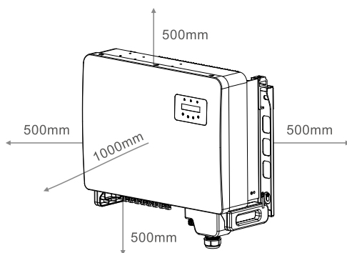
Rysunek 5.2 Obszar pomiędzy falownikiem a sąsiadującymi urządzeniami podczas montażu
