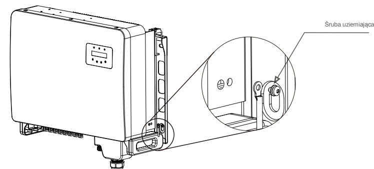
Rysunek 5.14 Kabel stały
