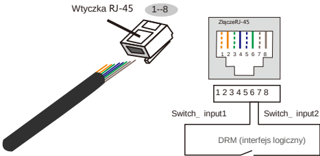
Rysunek 5.31 Zdjęcie warstwy izolacyjnej i podłączenie przewodu do wtyczki 3 RJ-45.Podłącz RJ-45 do interfejsu logicznego DRM.
