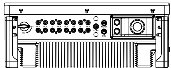
Rysunek 5.22 Podłączenie złącza prądu stałego do falownika
