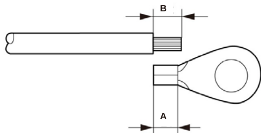
Rysunek 5.12 Odpowiednia długość
