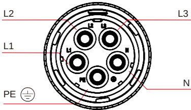
Rysunek 5.21 Konstrukcja wewnętrzna złącza prądu zmiennego
