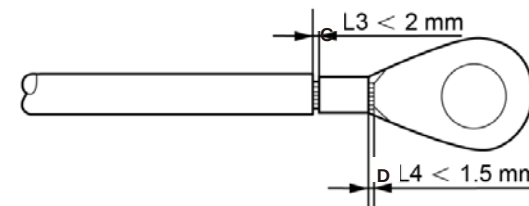
Rysunek 5.9 Przewód ze zdjętą izolacją
