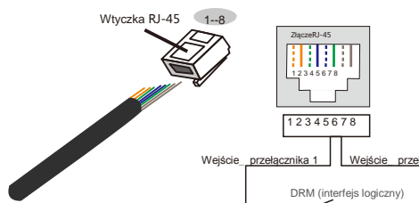
Rysunek 5.29 Zdjęcie warstwy izolacyjnej i podłączenie przewodu do wtyczki RJ-45
