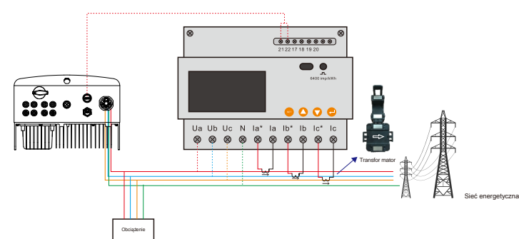
Rysunek 5.27 Podłączenie miernika (2)
