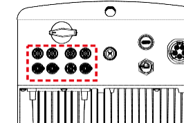
Rysunek 5.18 Podłączenie złącza prądu stałego do falownika
