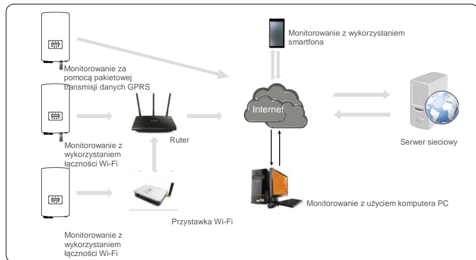
Rysunek 5.25 Funkcja komunikacji bezprzewodowej
