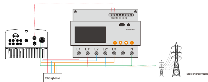
Rysunek 5.26 Podłączenie miernika (1)
